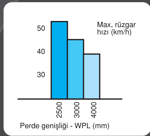
Rüzgar dayanım tablosu
